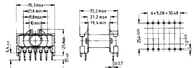
C-106. kép A 16 kivezetésű ETD-39 csévetest méretei
