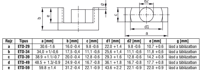
C-104. kép A 13 kivezetésű ETD-29 csévetest méretei
