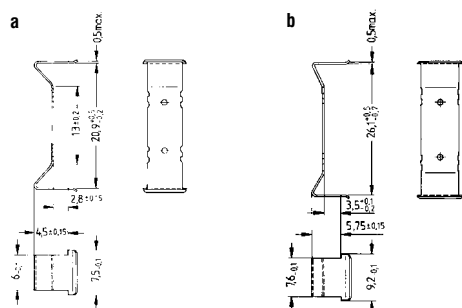
C-109. kép Az EF sorozatú kengyelek méretei
