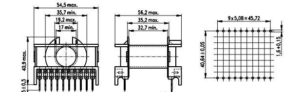
C-110. kép Az ETD-29, ETD-39 és ETD-49 kengyelek méretei
