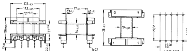
C-109. kép Az EF sorozatú kengyelek méretei
