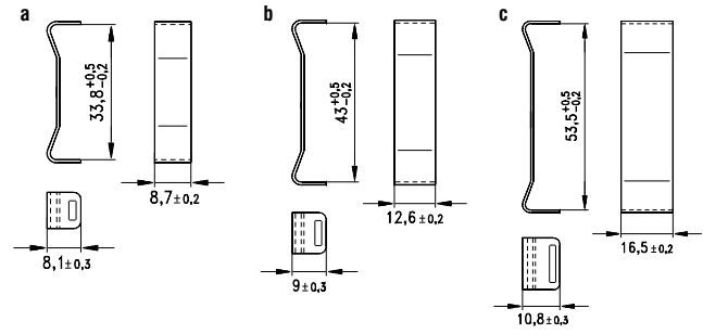
C-110. kép Az ETD-29, ETD-39 és ETD-49 kengyelek méretei
