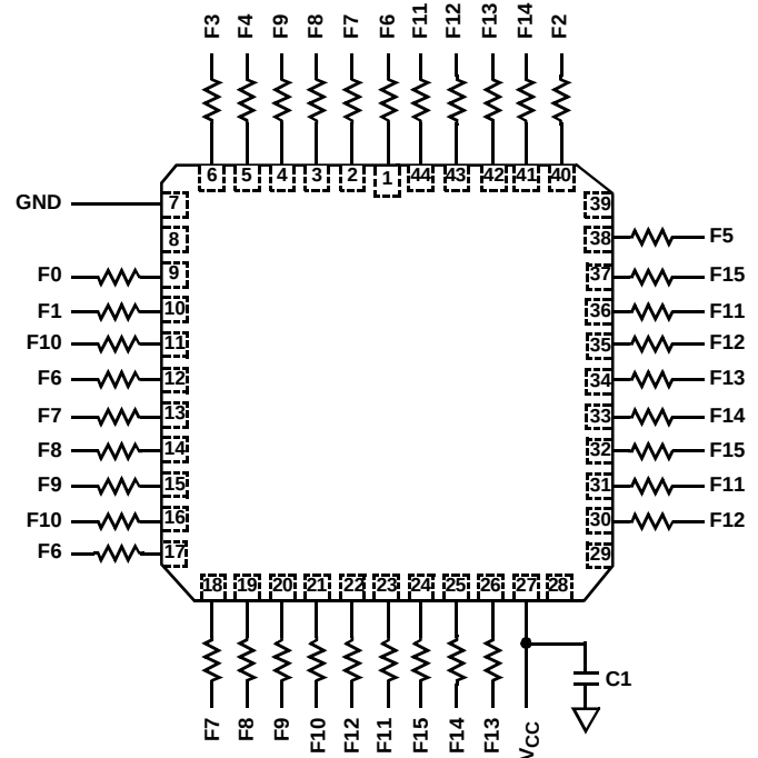
MR82C55A CLCC
