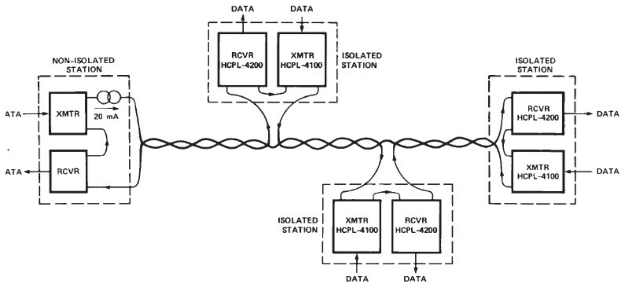
(b) MULTIDROP
