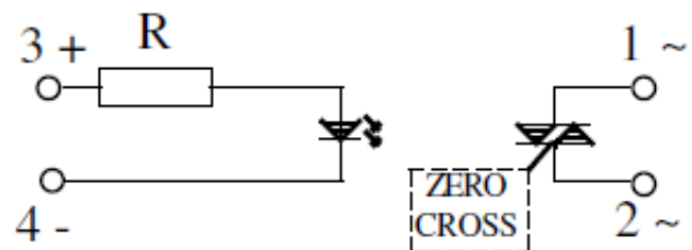
schéma équivalent / Equivalent circuit
