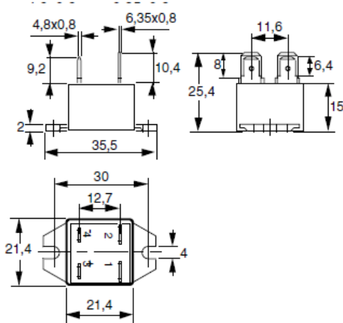
Modèle à cosses Fastons / Fastons connections model
