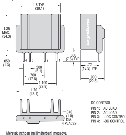
K-191. kép PF 240D25, PF 480D25 mérete
