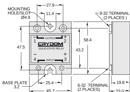
K-192. kép D1D20, D1D40 méretei
