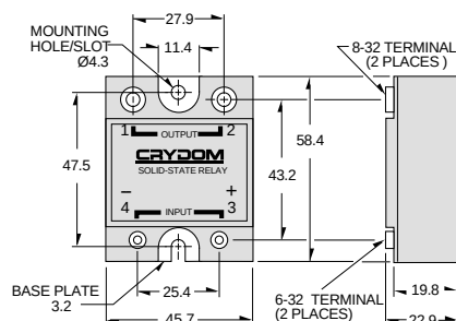
K-190. kép D53TP50D mérete
