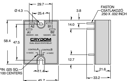
K-189. kép D2440D mérete
