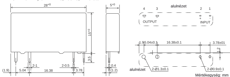
FTR-SL PK012W, OPT-24DC/230AC/1 méretei
