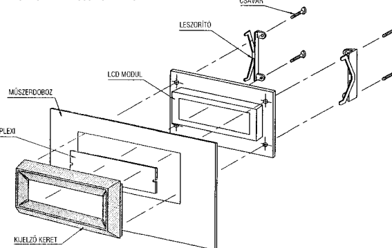
DISPLAY KIJELZŐ KERETEK ÖSSZESZERELÉSE
