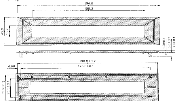
DISPLAY KIJELZŐ KERETEK ÖSSZESZERELÉSE
