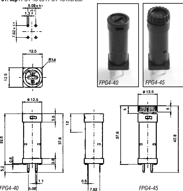
M-81. kép FPG4-40 és FPG4-45 méretei
