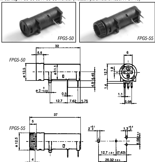
M-82. kép FPG5-50 és FPG5-55 méretei (műszaki paraméterek lásd. FPG4-40)
