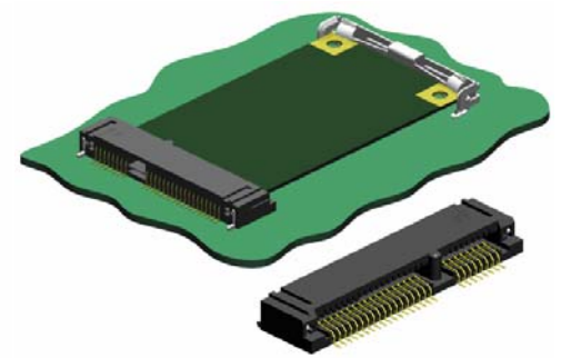
Mini PCI Express Connectors
