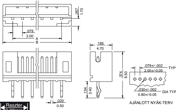
L-325. kép EGYENES BEÜLTETHETŐ TŰSKESOR
