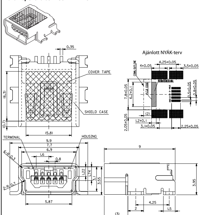
L-649. kép 54819-0572 USB-B MINI SMD
