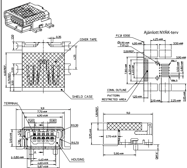
L-648. kép 67503-1020 USB-B MINI SMD
