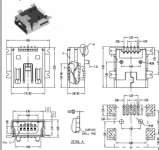
L-651. kép 65100516121 USB-B MINI SMD
