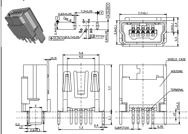
L-650. kép 500075-1517 ÁLLÓ USB-B MINI SMD
