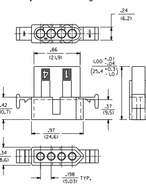
L-376. kép 03-09-2041 dugó
