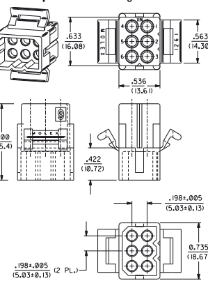
L-378. kép 03-09-2061 dugó
