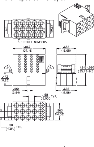
L-379. kép 03-09-1151 aljzat
