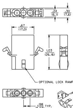
L-373. kép 03-09-1031 aljzat
