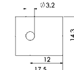
M-245. kép TO-220-ALU szilikon méretei
