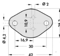
M-240. kép TO-3-FIS szilikon méretei
