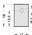
M-240. kép TO-3-FIS szilikon méretei
