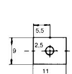
M-243. kép TO-126 szilikon méretei
