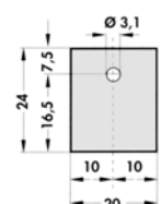
M-241. kép TOP-3-FIS szilikon méretei
