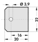
M-241. kép TOP-3-FIS szilikon méretei
