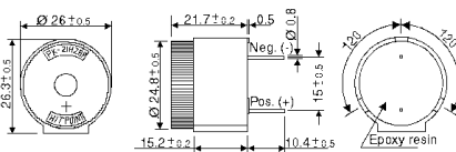
N-88. kép ZÜMMER PIEZO PK 21H28PQ
