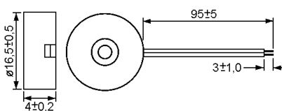
N-89. kép ZÜMMER PIEZO-LAP PT 1550WQ
