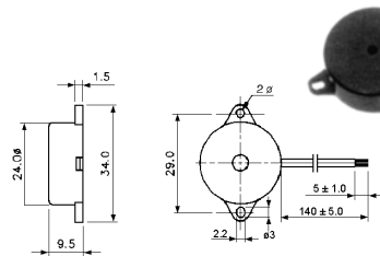
N-89. kép ZÜMMER PIEZO-LAP PT 1550WQ
