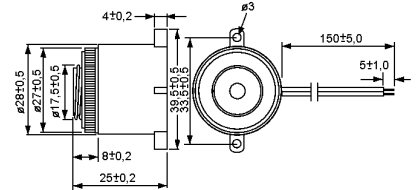
N-90. kép ZÜMMER PIEZO-LAP PT1340PP10PQ
