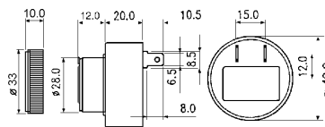
N-88. kép ZÜMMER PIEZO PK 21H28PQ
