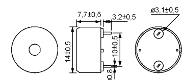
N-90. kép ZÜMMER PIEZO-LAP PT1340PP10PQ
