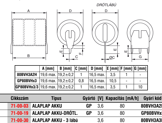
0-254. kép 80BVH3A2H és GP80BVHx3 méretei
