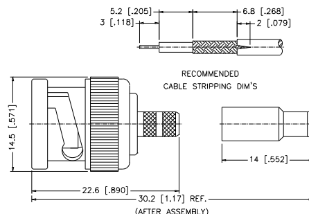
L-501. kép KRIMPELHETŐ LENGŐ DUGÓ
