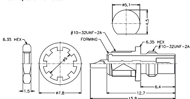
L-499. kép 83-02-44 méretei
