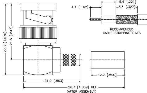
L-502. kép 90°-OS KRIMPELHETŐ LENGŐ DUGÓ
