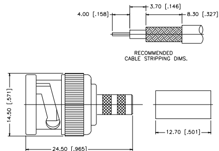
L-500. kép KRIMPELHETŐ LENGŐ DUGÓ
