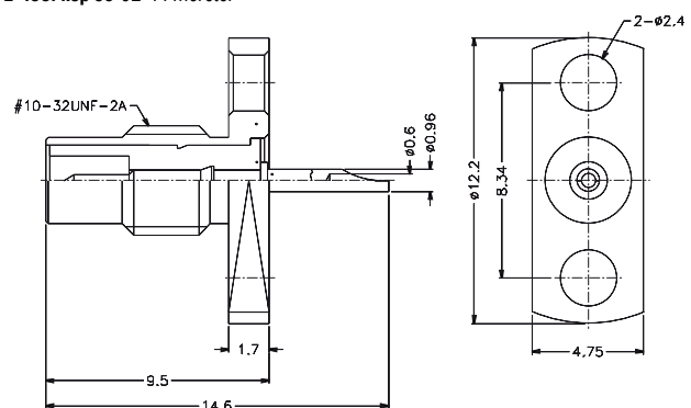
L-499. kép 83-02-44 méretei
