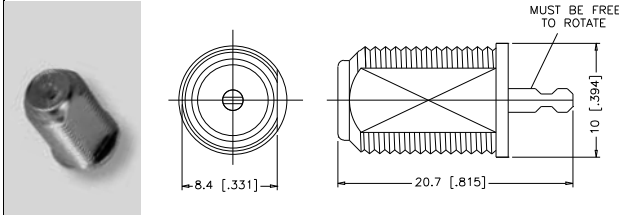
L-527. kép SZERELHETŐ ALJZAT
