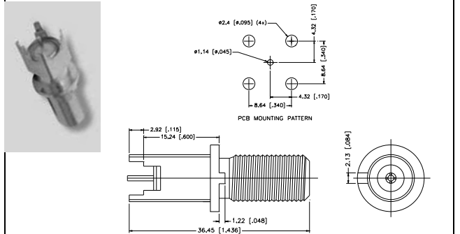
L-530. kép NYÁKBA ÜLTETHETŐ EGYENES ALJZAT
