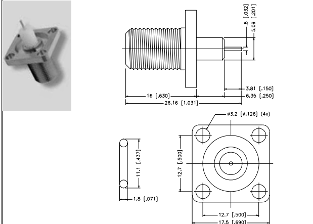
L-528. kép 4 CSAVARRAL ELŐLAPRA SZERELHETŐ FORRASZTHATÓ ALJZAT
