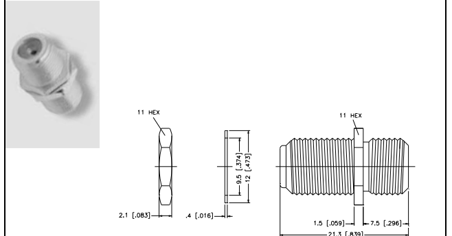
L-531. kép TOLDÓ ALJZAT-ALJZAT
