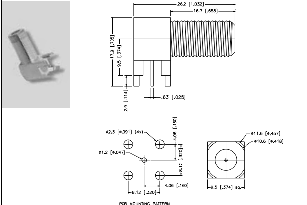
L-529. kép NYÁKBA ÜLTETHETŐ 90°-OS ALJZAT
