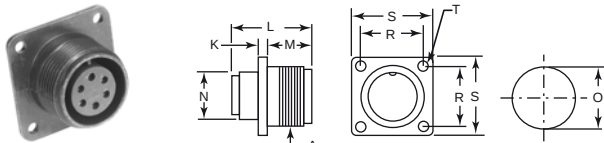
L-770. kép MS 3102A és MS 3102E sorozatú csatlakozók méretei
