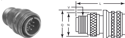
L-771. kép MS 3106A sorozatú csatlakozók
