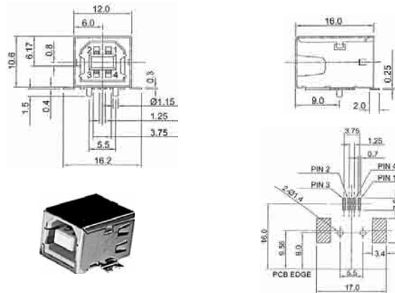
L-643. kép 90°-os USB-BSMT aljzat NYÁK-ba
