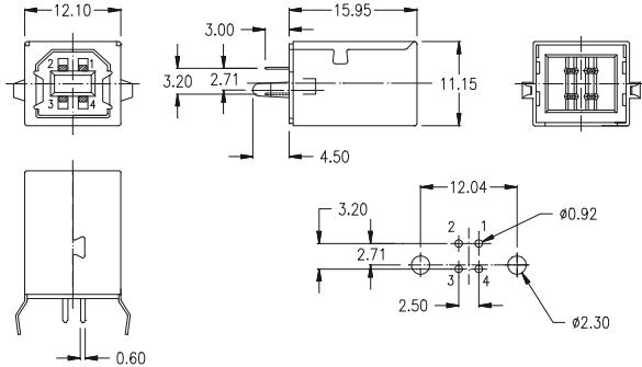
L-645. kép USB-B csatlakozó
