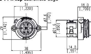
L-715. kép Szerelhető aljzat
