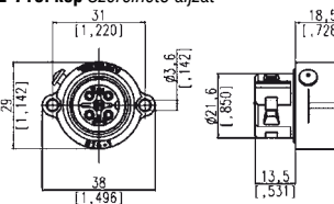
L-715. kép Szerelhető aljzat
