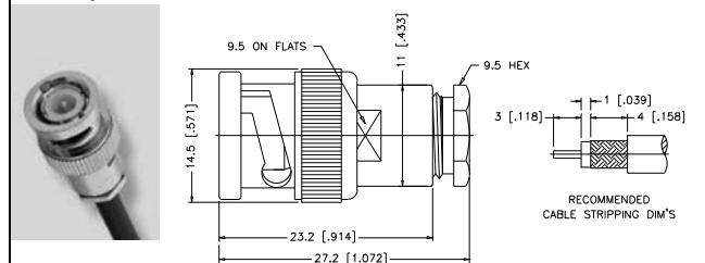
L-507. kép SZERELHETŐ LENGŐ DUGÓ
