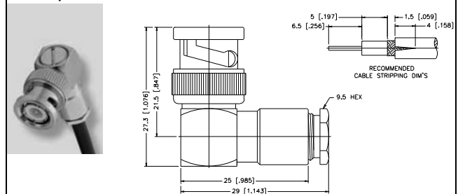
L-508. kép 90°-OS SZERELHETŐ LENGŐ DUGÓ
