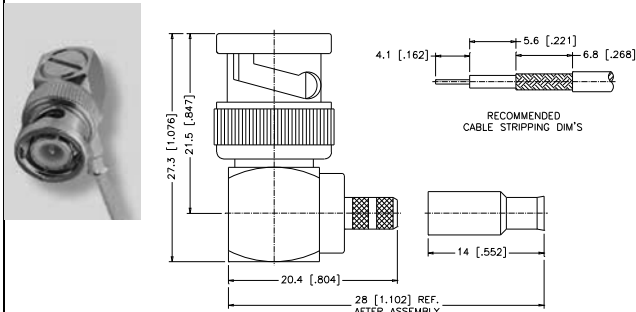
L-503. kép 90°-OS KRIMPELHETŐ LENGŐ DUGÓ VÉkony KÁBELHEZ
