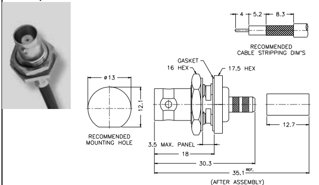
L-505. kép ELŐLAPRA SZERELHETŐ KRIMPELHETŐ ALJZAT
