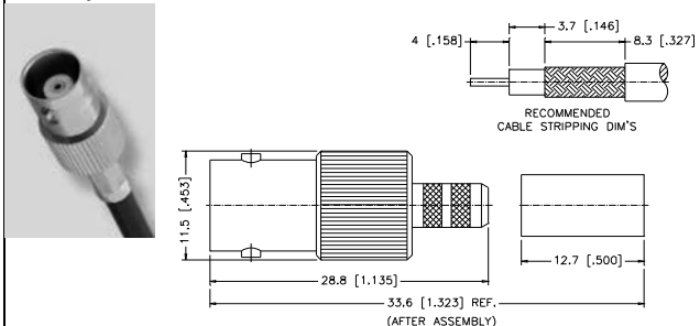
L-504. kép KRIMPELHETŐ LENGŐ ALJZAT
