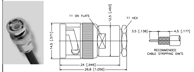
L-506. kép SZERELHETŐ LENGŐ DUGÓ VÉkony KÁBELHEZ
