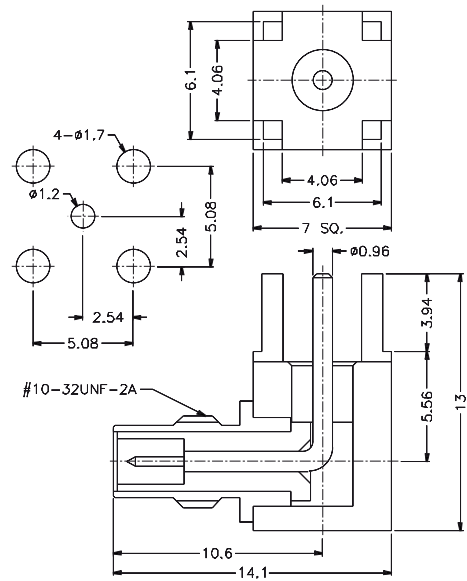
L-495. kép 83-02-42 méretei
