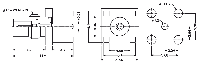
L-495. kép 83-02-42 méretei
