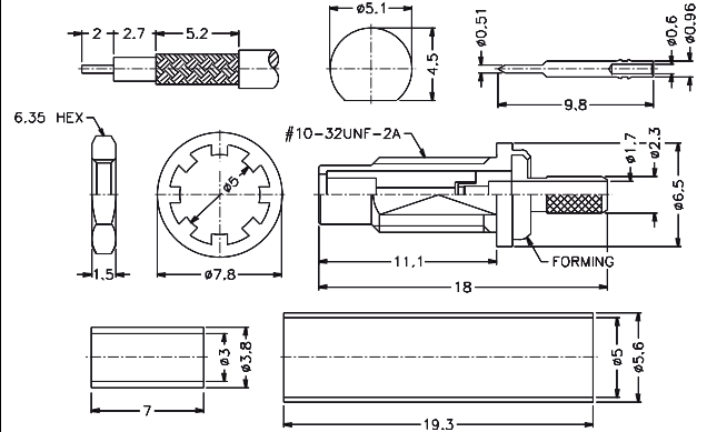
L-494. kép 83-02-41 méretei
