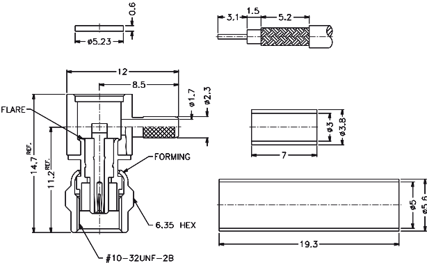
L-489. kép 83-02-40, 83-05-01 méretei
