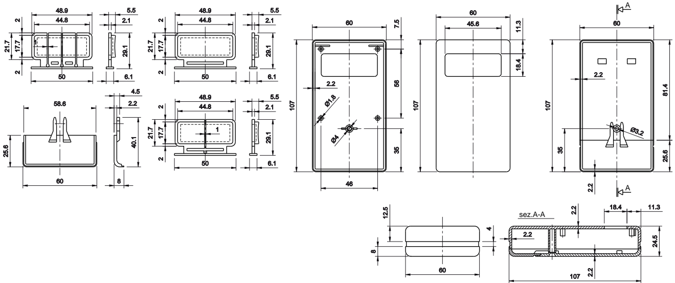
N-162. kép TEKO RC124.5, TEKO RC124.9
