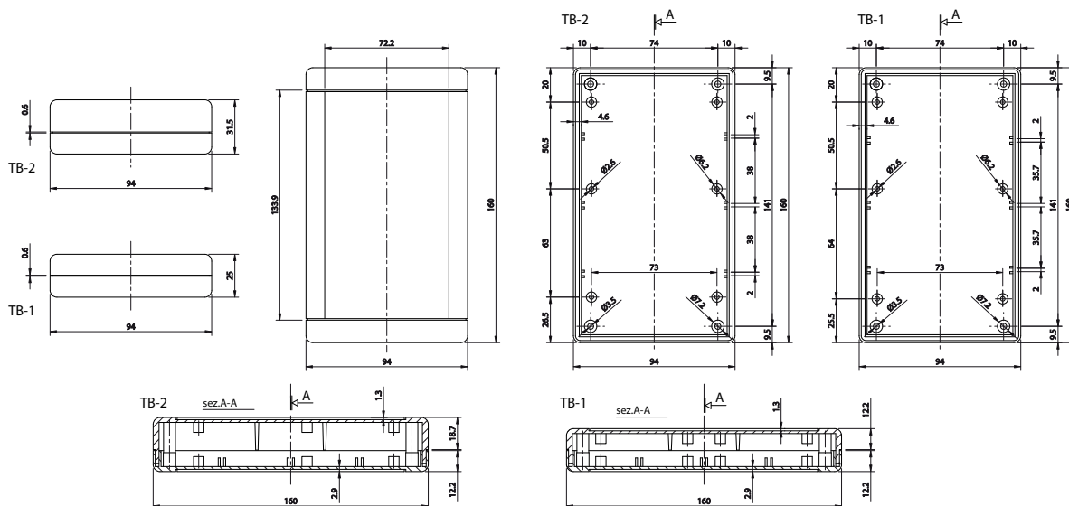
N-184. kép TEKO TB-1.7, TEKO TB-1.9, TEKO TB-2.7, TEKO TB-2.9
