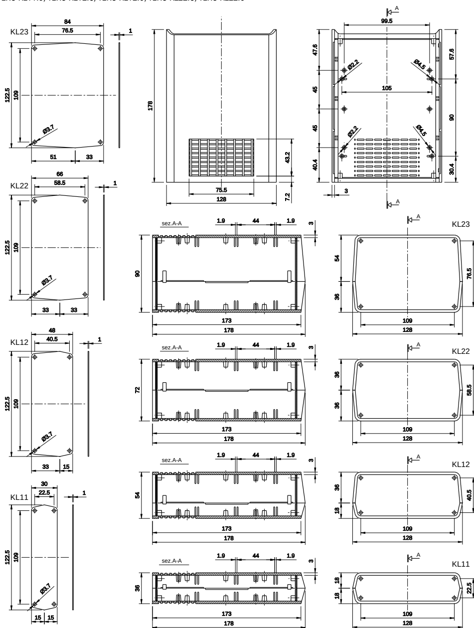
N-273. kép TEKO KL11.5, TEKO KL11.9, TEKO KL12.5, TEKO KL12.9, TEKO KL22.5, TEKO KL22.9
