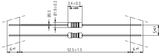
A-1. kép A CFR25S (0204) méretei
