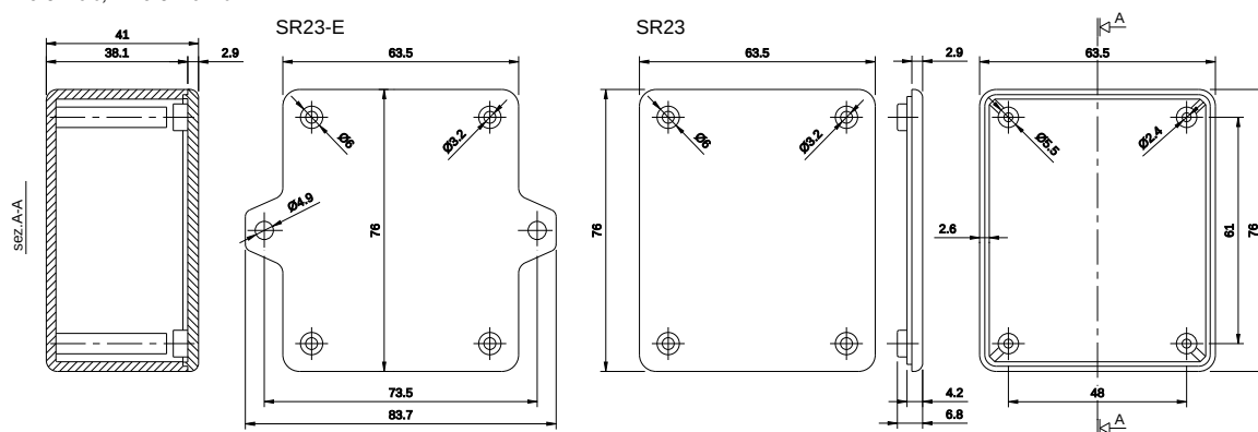
N-194. kép TEKO SR23.9, TEKO SR23-E.9
