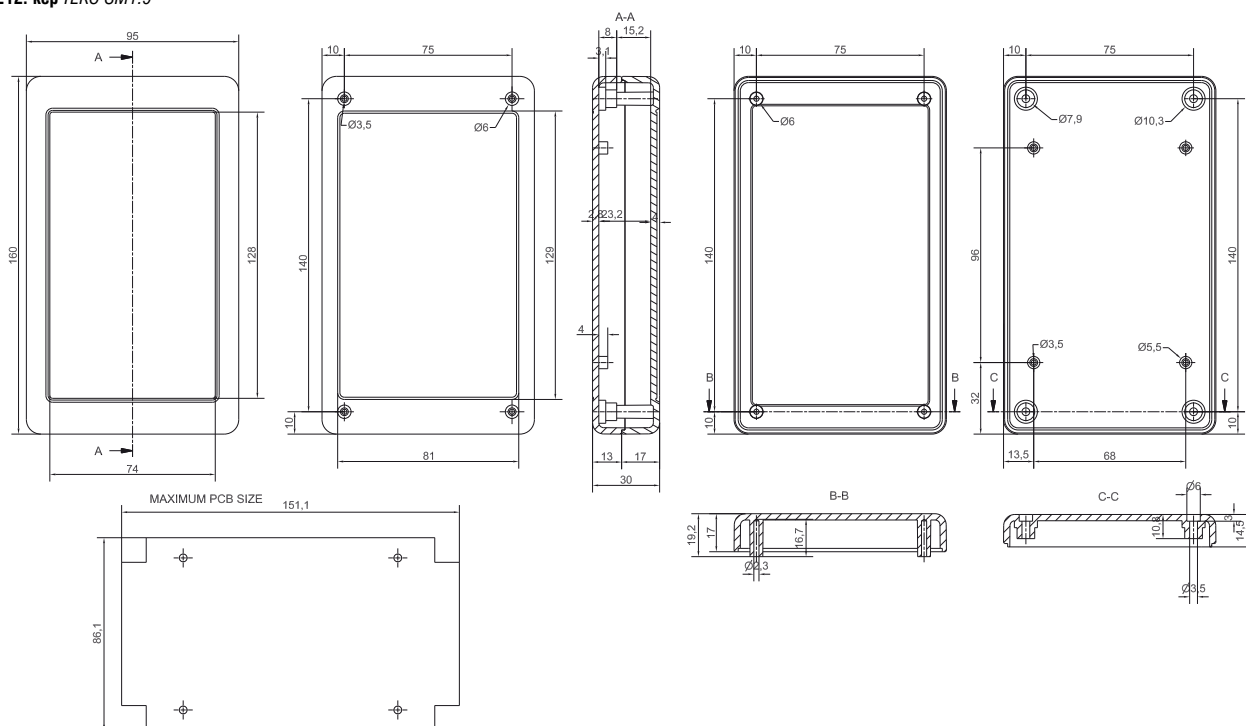
N-213. kép TEKÓ SM-B.7, TEKÓ SM-B.9, TEKÓ SMS-B.7, TEKÓ SMS-B.9
