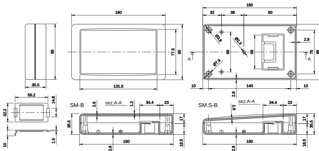
N-213. kép TEKÓ SM-B.7, TEKÓ SM-B.9, TEKÓ SMS-B.7, TEKÓ SMS-B.9
