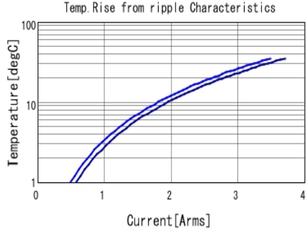
GRM188R6YA225KA12 Temp. rise ■ 500kHz ■ 1MHz
