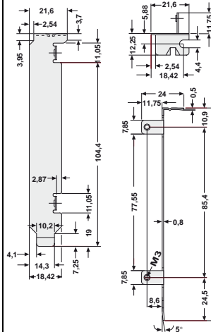
N-425. kép PCI...L
