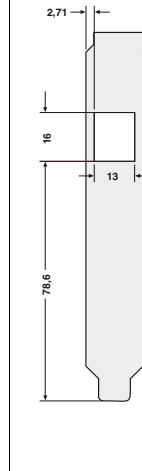
N-427. kép PCI 027L
