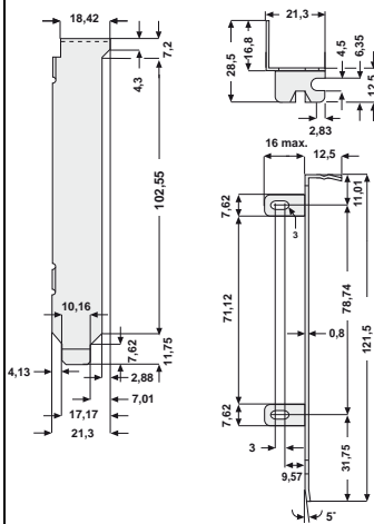
N-423. kép KHPC...L felerősítő fülekkel
