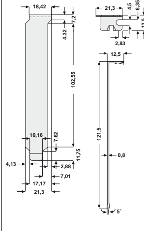
N-424. kép KHPC...O felerősítő fülek nélkül
