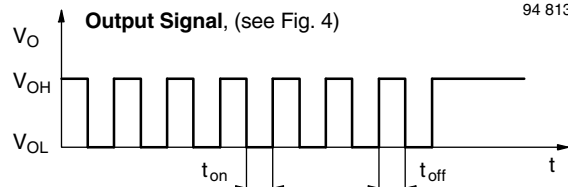
Fig. 3 - Output Function
