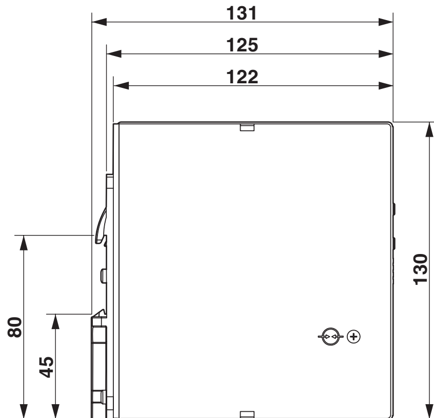
Méretrajz
