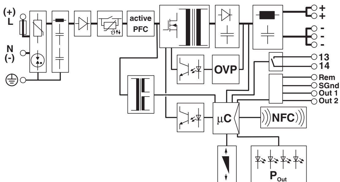
Blokkvázlat
