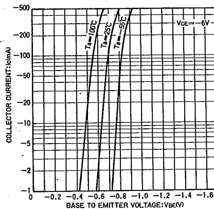
Fig.2 エミッタ接地伝達特性
