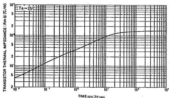
Fig.11 過渡熱抵抗
