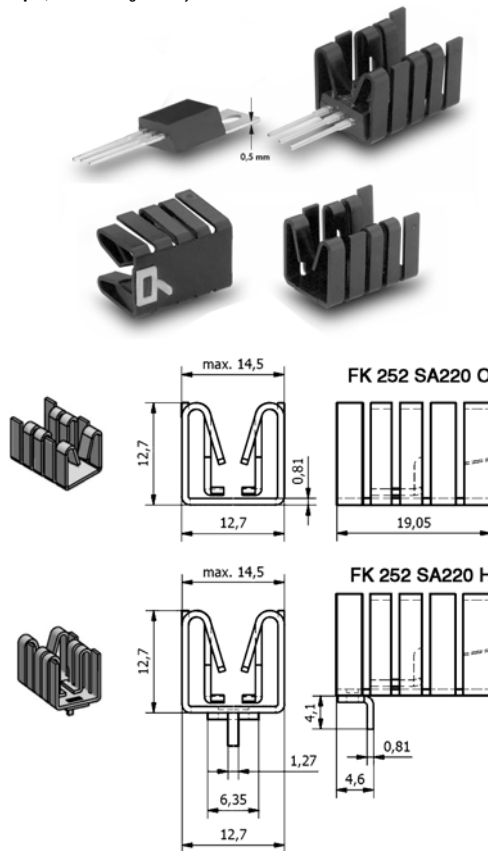
M-138. kép 0,5mm vastag zászlójú TO-220 tokozásokhoz
