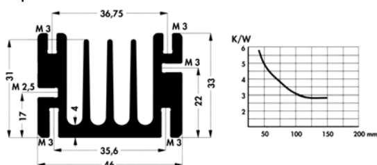
M-221. kép SK 68 méretei
