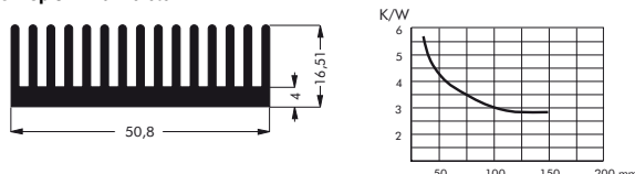
M-223. kép SK 426 méretei
