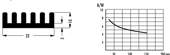
M-219. kép SK 400 méretei
