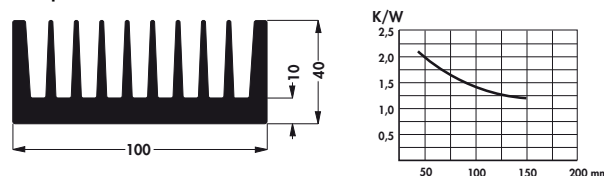
M-226. kép SK 92 méretei
