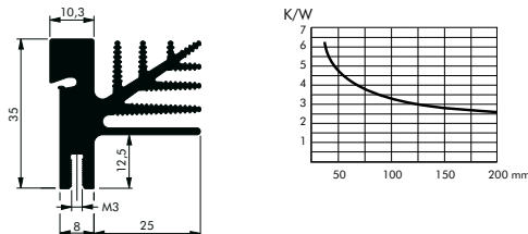
M-220. kép SK 482 méretei
