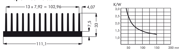
M-227. kép SK 433 méretei
