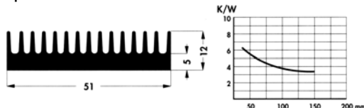
M-224. kép SK 156 méretei
