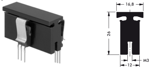
M-217. kép SK 492 méretei
