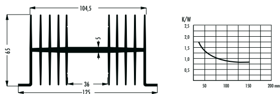
M-228. kép SK 34 méretei
