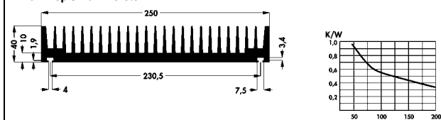
M-232. kép SK 91 méretei
