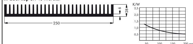
M-233. kép SK 49 méretei
