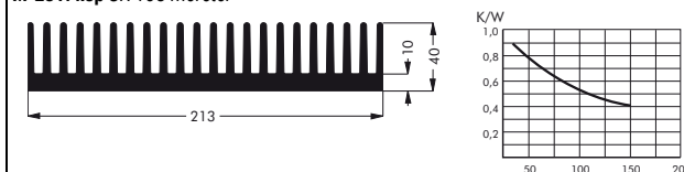
M-231. kép SK 193 méretei
