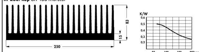
M-235. kép SK 438 méretei
