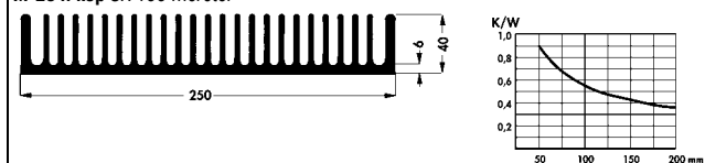
M-234. kép SK 199 méretei
