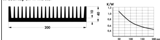
M-230. kép SK 47 méretei
