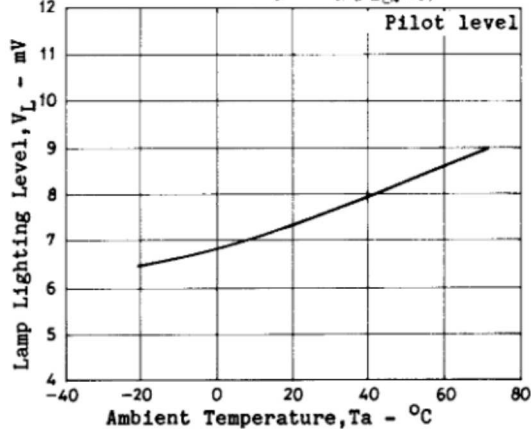
V_L - T_a (Fig. 25)
